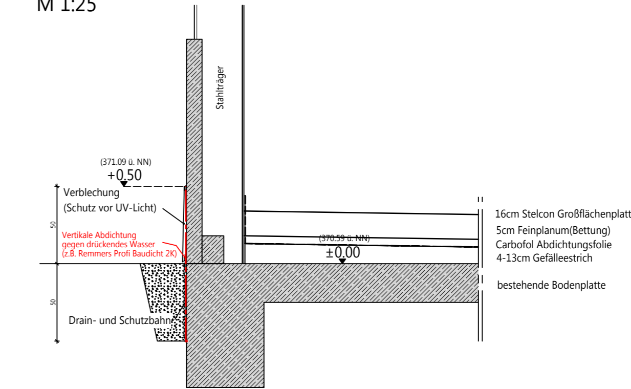
Sockelanschluß aussen gegen drückendes Wasser M 1:25
