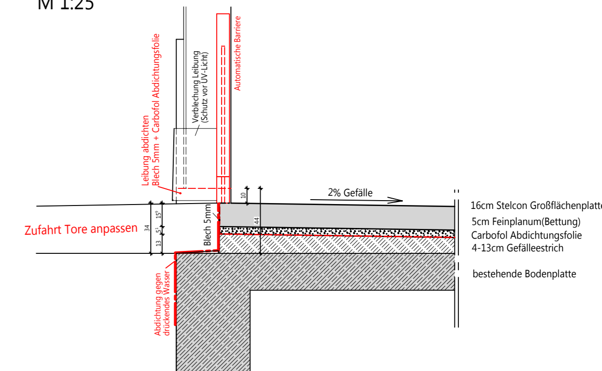
Sockelanschluß-Türbereich M 1:25
